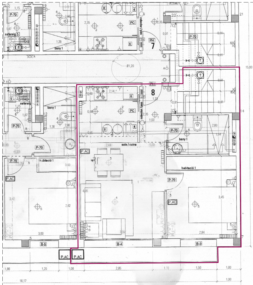
PLANTA SEGONA
